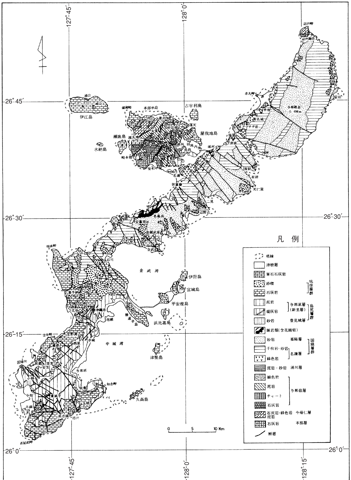
第6図 沖縄本島の地質図
